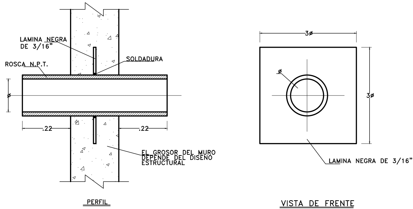
DETALLE TÍPICO NIPLE PASAMUROS SIN ESCALA
