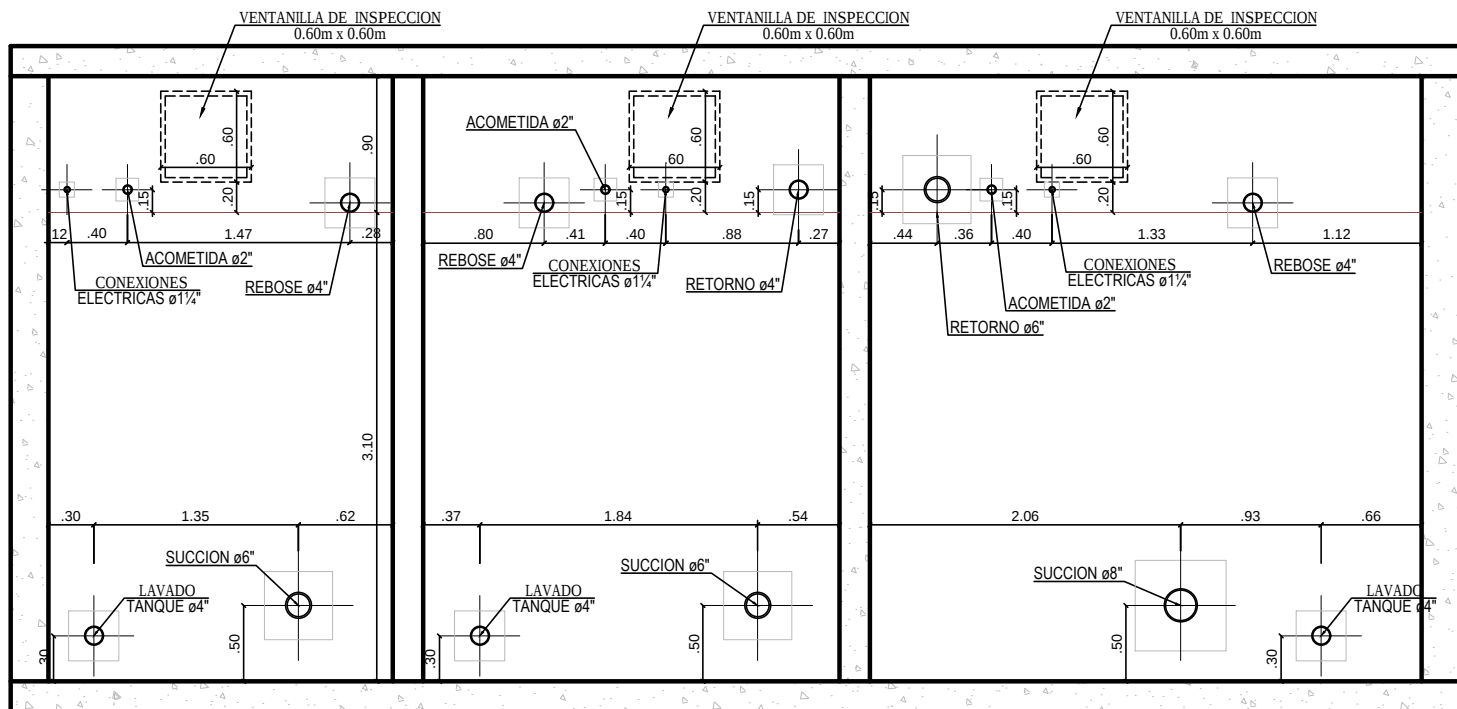
DETALLE NIPLES PASAMUROS CUARTO DE BOMBAS AGUA POTABLE Y RED CONTRA INCENDIO ESCALA 1:50
