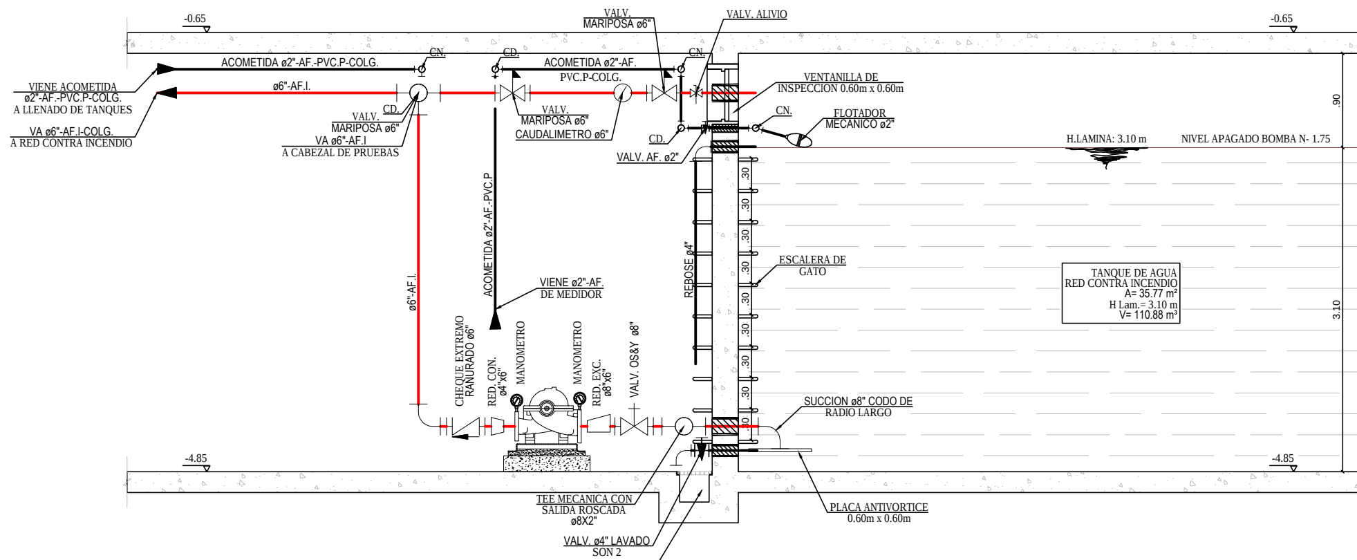
DETALLE CORTE B-B' CUARTO DE BOMBAS RED CONTRA INCENDIO ESCALA 1:50
