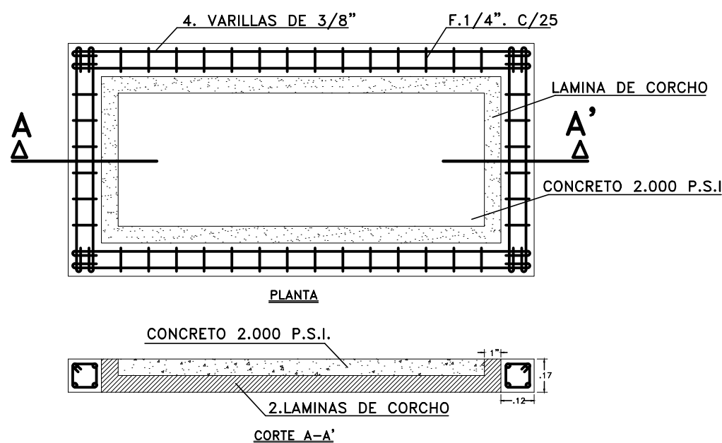
DETALLE BASE ANTIVIBRATORIA SIN ESCALA
