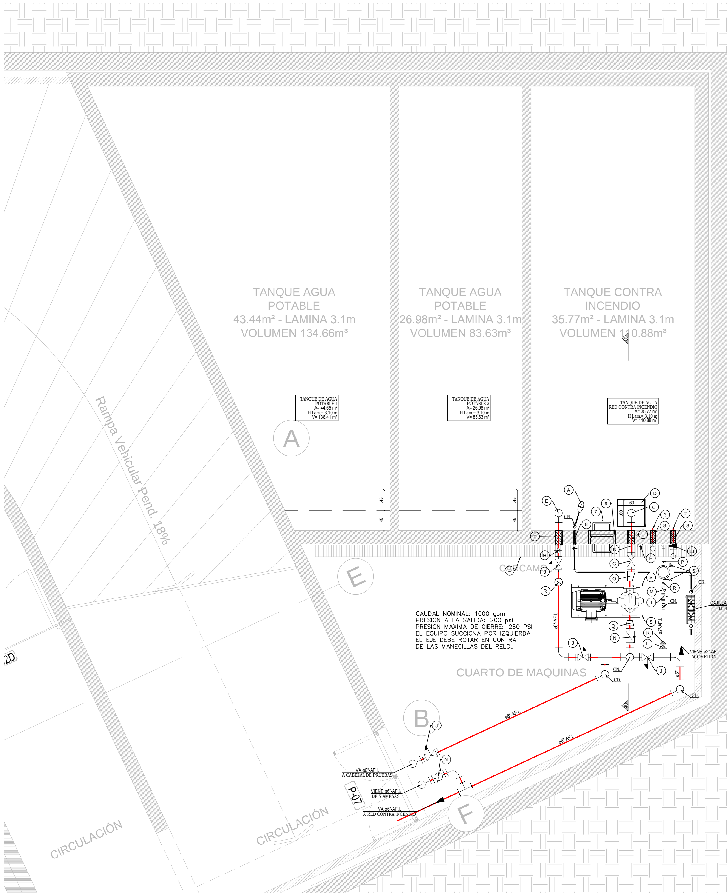
DETALLE CUARTO DE BOMBAS RED CONTRA INCENDIO ESCALA 1:50
