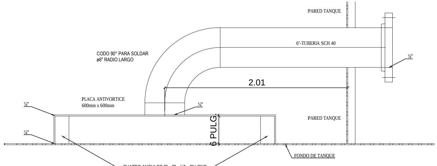
DETALLE PLACA ANTIVORTICE SIN ESCALA
